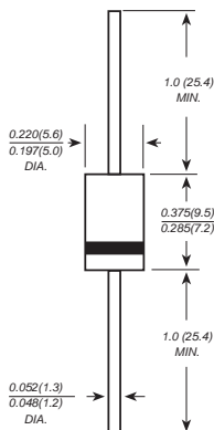
DO-201AD
